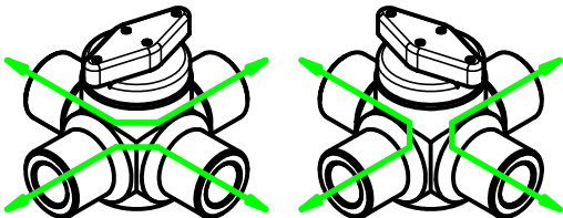
4-Wege mit Doppel-L-Bohrung
