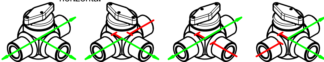
3-Wege mit T-Bohrung, horizontal
