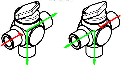
3-Wege mit Winkelbohrung, vertikal
