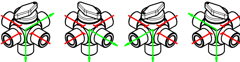
5-Wege mit Winkelbohrung
