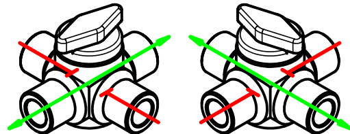
4-Wege mit Durchgangsbohrung
