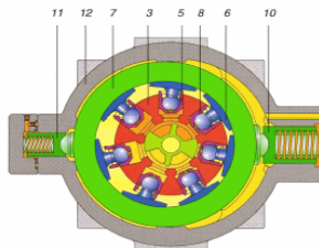
Vereinfachte Darstellung des Aufbaus der RKP-Pumpen
